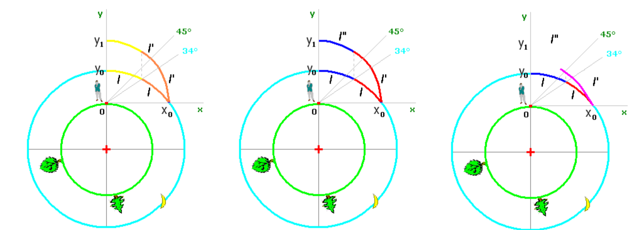
Obr. 3 26-nova-vyska-Mesice.PNG
