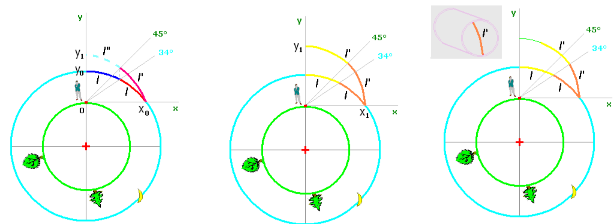
Obr. 3 26-nova-vyska-Mesice.PNG
