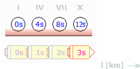
Obr. 17. Prostorové vjemy pozorovatele na podsvětelném korábu skládají výsledný zážitek geometrické délky (v pohybu, 4 fáze)
