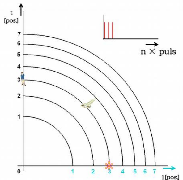
Obr. 11. Zdroj pulsů určuje pohyb ve spojitým perspektivním časoprostoru ( v pohybu, 10 fází )
