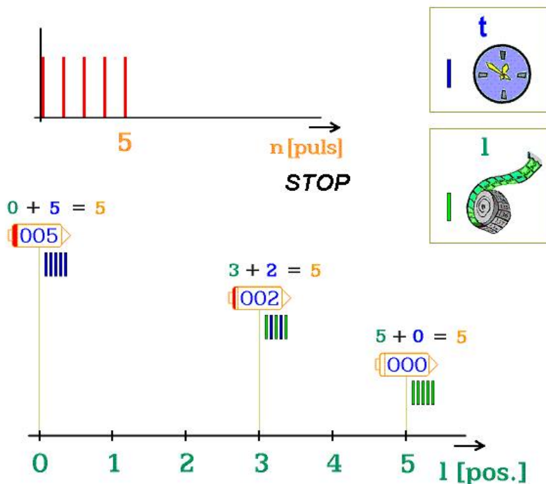
Obr. 15. Tři hvězdolety, o ustálených rychlostech, v posicích prostoru ( v pohybu, 11 fázi )
